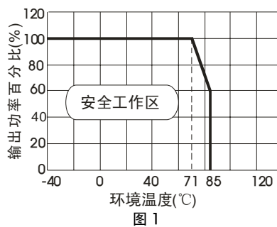
温度降额曲线
