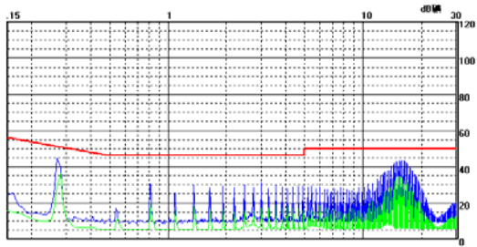
WRB1205S-3WR2 传导骚扰 Class B 测试效果图 (正线)
