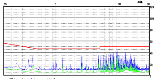
WRA2415S-3WR2 传导骚扰 Class B 测试效果图 (负线)
