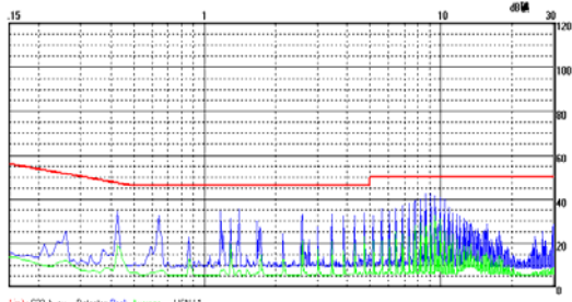
WRA2415S-3WR2 传导骚扰 Class B 测试效果图 (正线)
